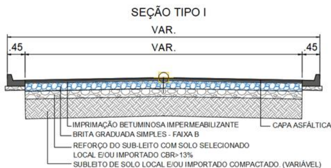
Figura 1 - Estrutura do pavimento
